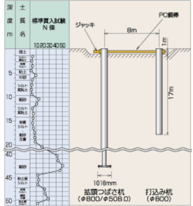
粘性土地盤での試験
